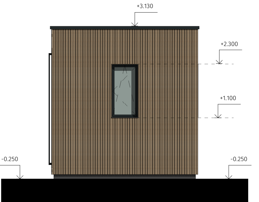
Pohľad severný M 1:100
