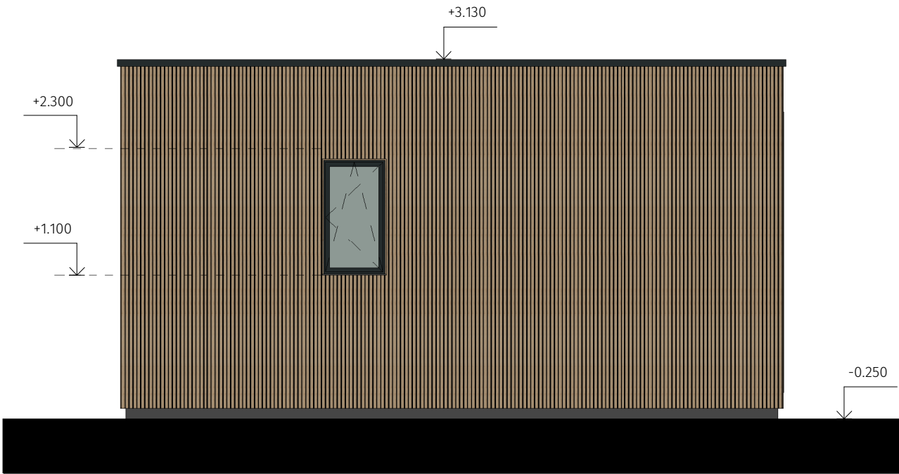
Pohľad východný M 1:100
