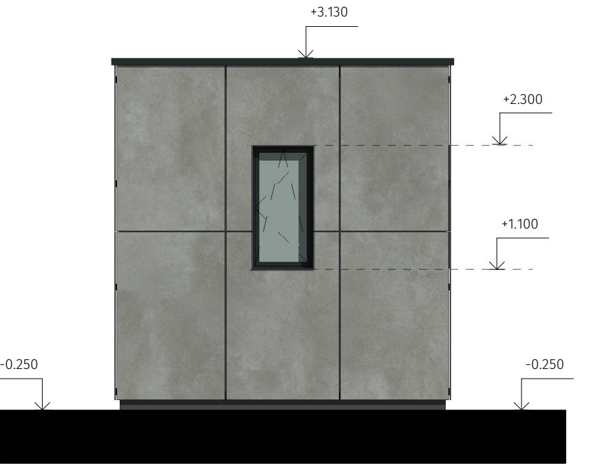
Pohľad severný M 1:100
